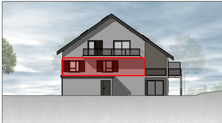
Élévation Sud-Est
